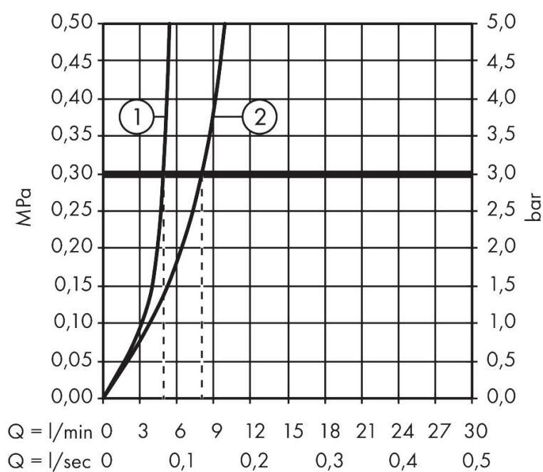
流量図
